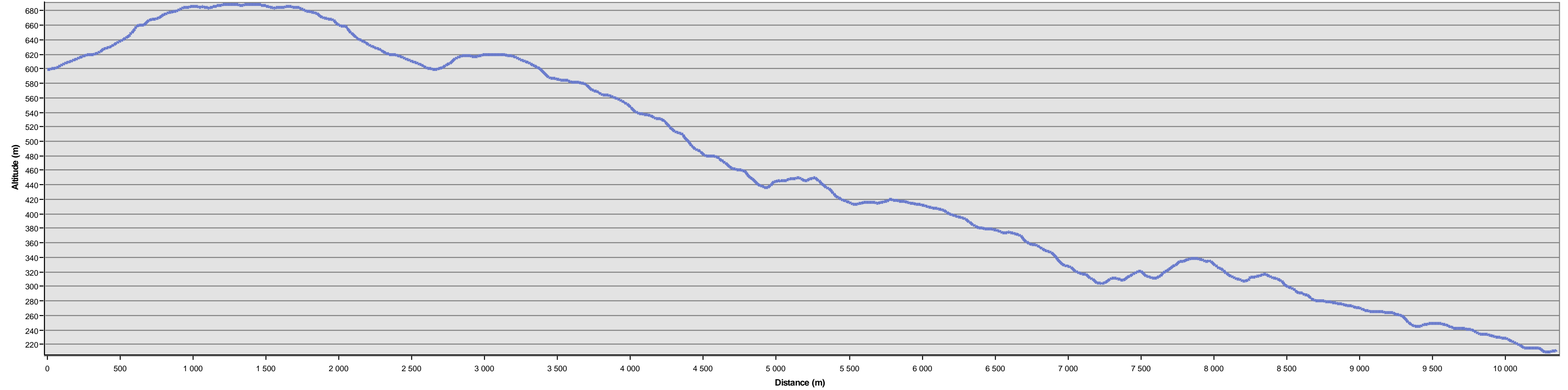
Coupe topographique - Parcours 10 km (UTCC)
