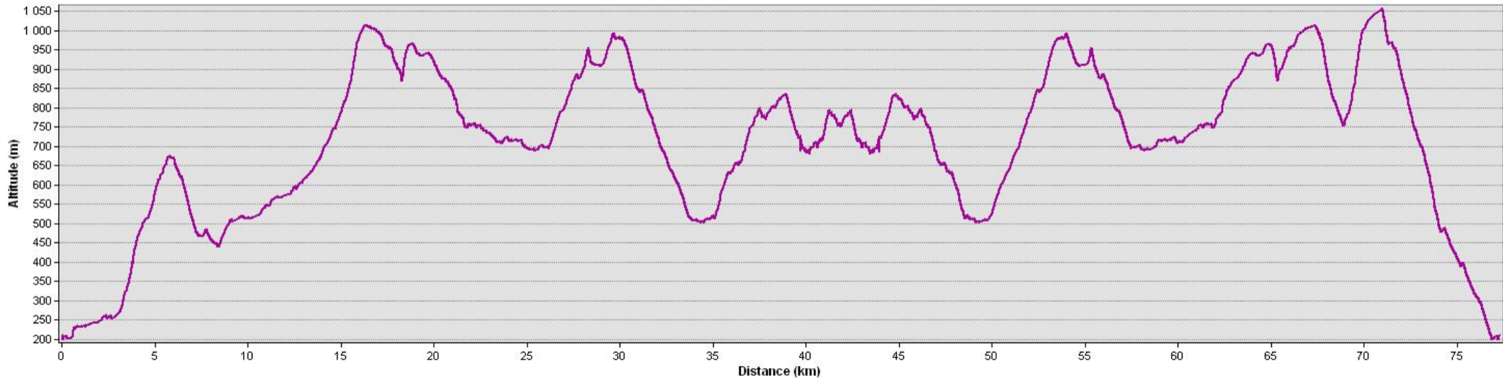
Coupe topographique - Parcours 78 km (UTCC)
